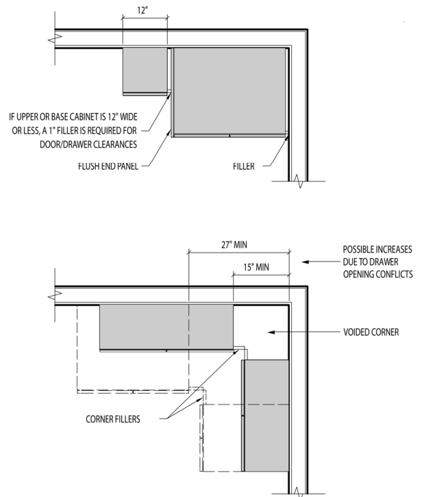
4 PLAN - FILLERS SCALE: RE:
